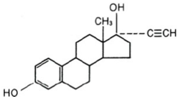
Ethinyl Estradiol C_{20}H_{24}O_2 MW: 296.4
