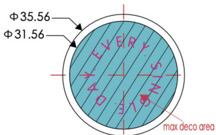
CAP MAX DECO AREA 盖顶部最大印刷区域
