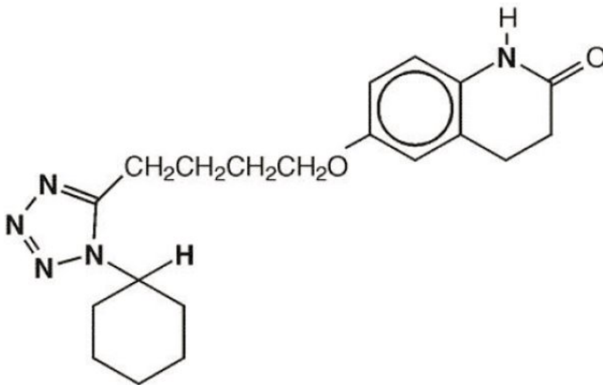
CILOSTAZOL
