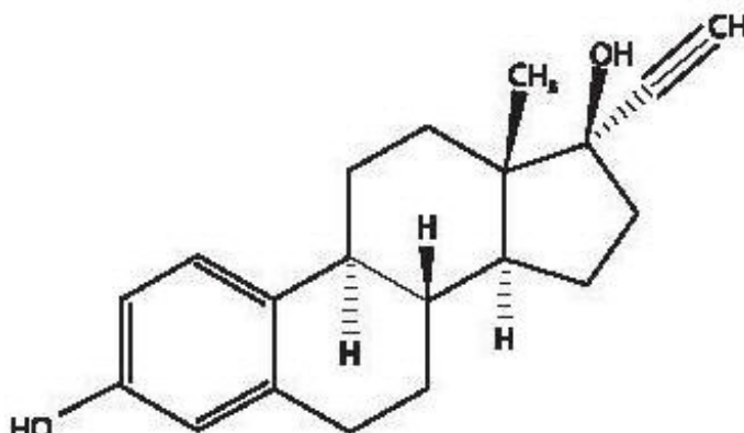
Ethinyl Estradiol
