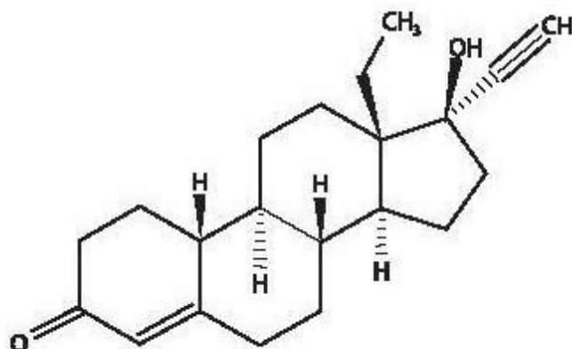
Levonorgestrel
