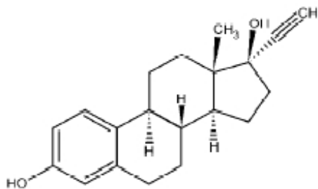
Ethinyl Estradiol C_{20}H_{24}O_2
