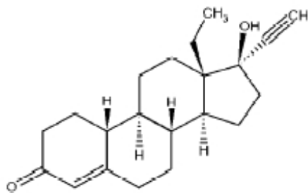
Levonorgestrel C_{21}H_{28}O_2
