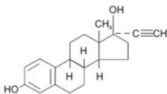
Ethinyl Estradiol
