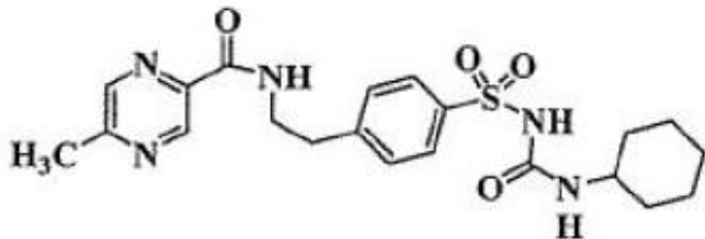
Glipizide
