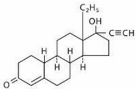
Levonorgestrel C 21 H 28 O 2 M.W. 312.45
