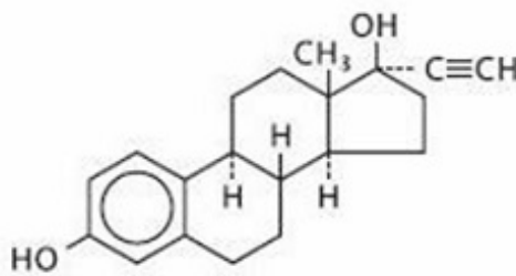
Ethinyl Estradiol C 20 H 24 O 2 M.W. 296.4
