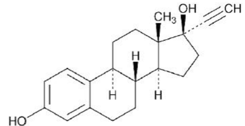
Ethinyl Estradiol
