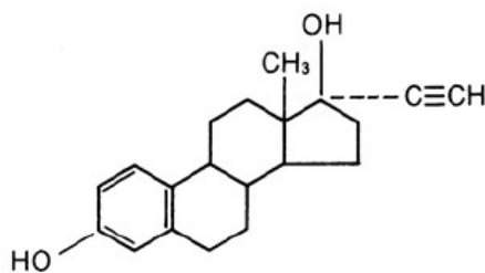
Ethinyl Estradiol
