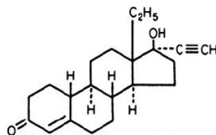
Levonorgestrel
