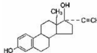
Ethinyl estradiol
