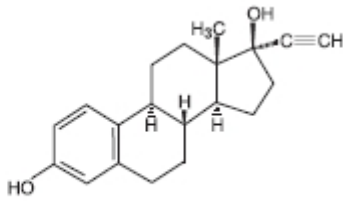
Ethinyl estradiol
