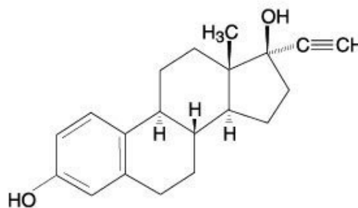
Ethinyl estradiol
